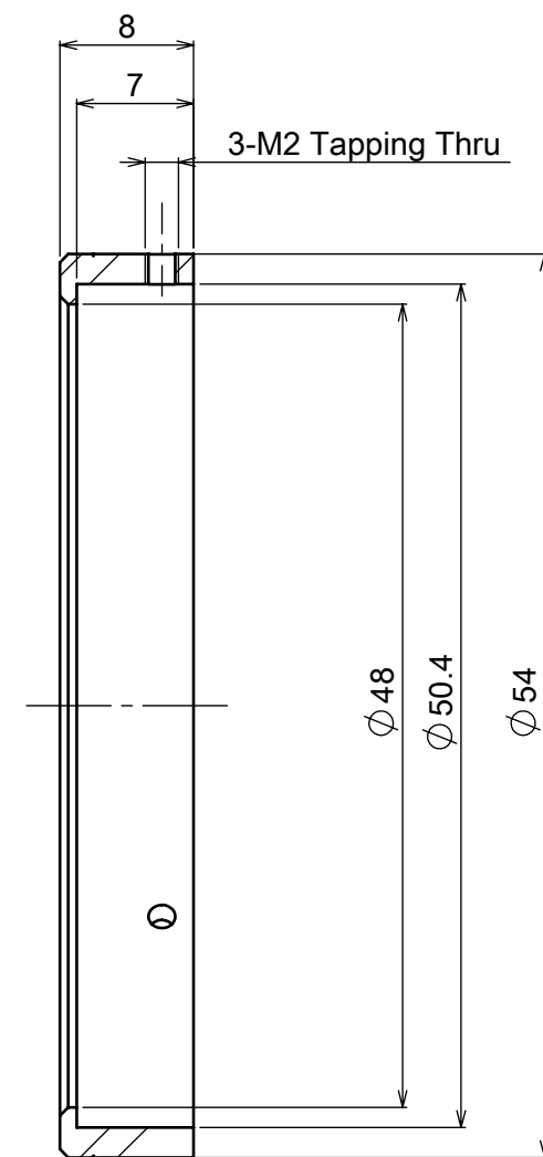
SECTION A-A
